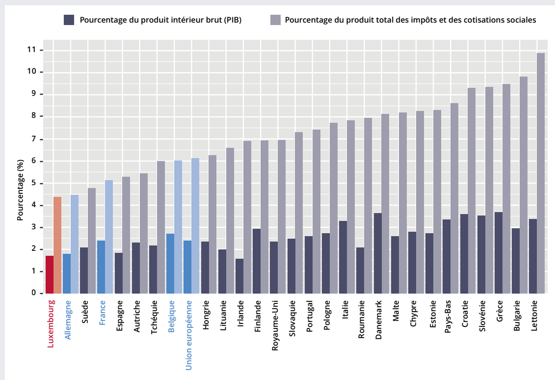
Graphique 4 : Revenus des taxes environnementales en Europe (2018)
