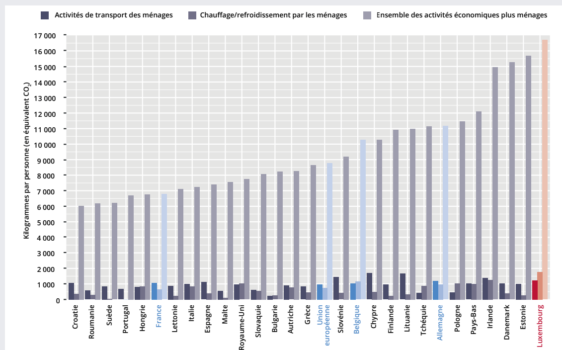
Graphique 1 : Émission de gaz à effet de serre par personne en Europe, 2018
